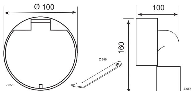
Prise d'aspiration au sol DISAN, avec couvercle de protection et microinterrupteur
